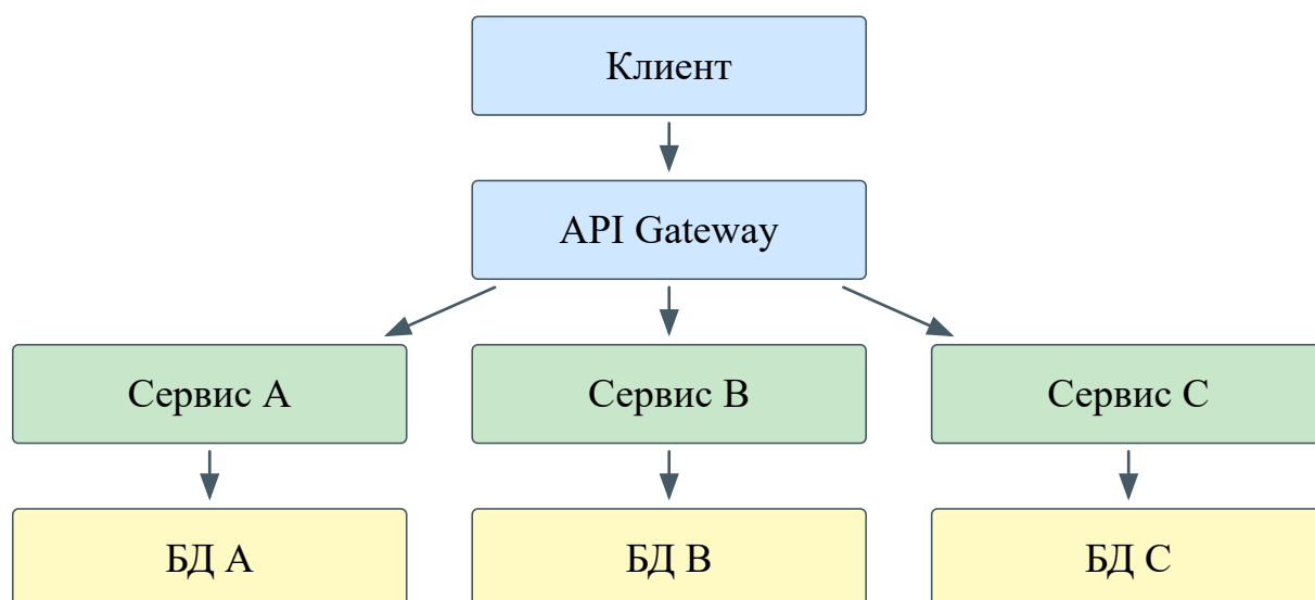
Рис. 8. Микросервисная архитектура
